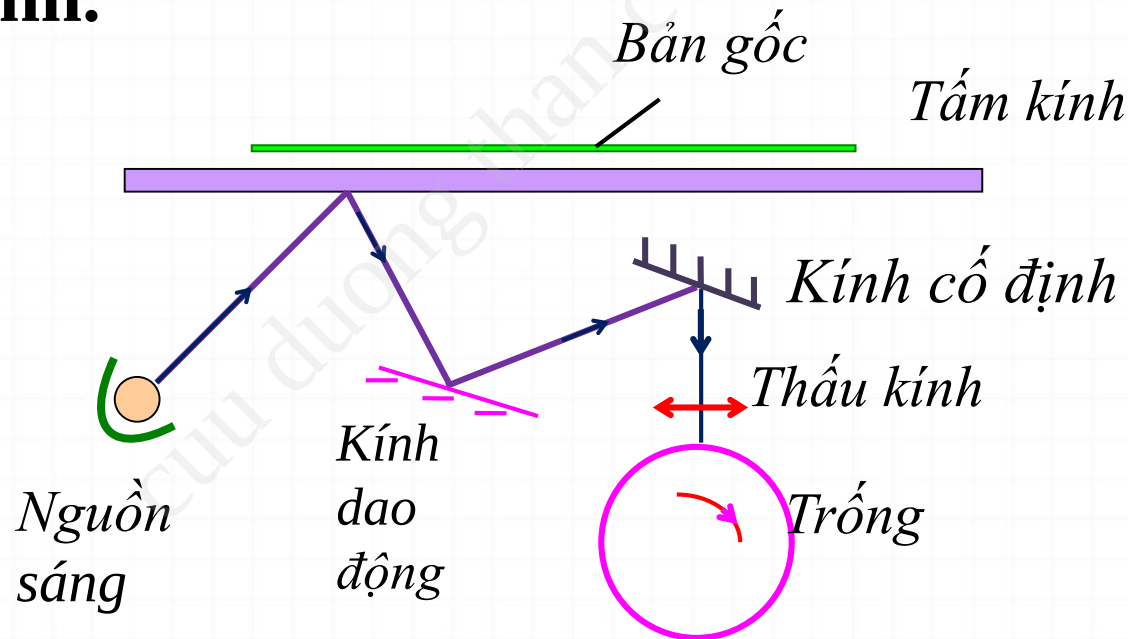
Sơ đồ máy photocopy
