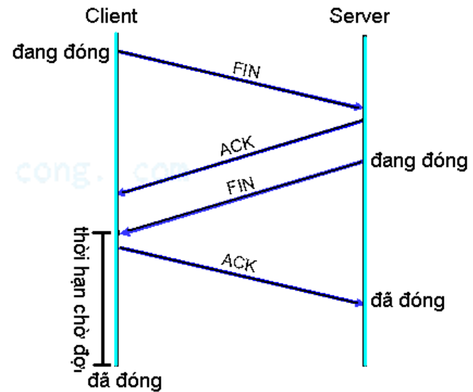
Hủy bắt tay trong TCP
