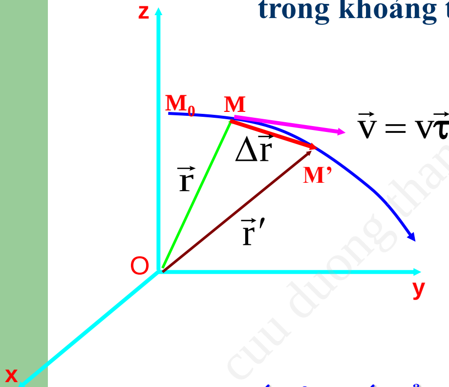
Hình 1.4: Vận tốc của chất điểm
