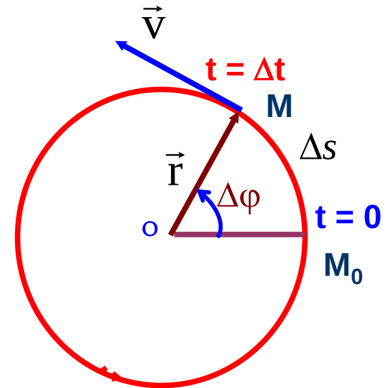
Hình 1.7: Vận tốc góc
