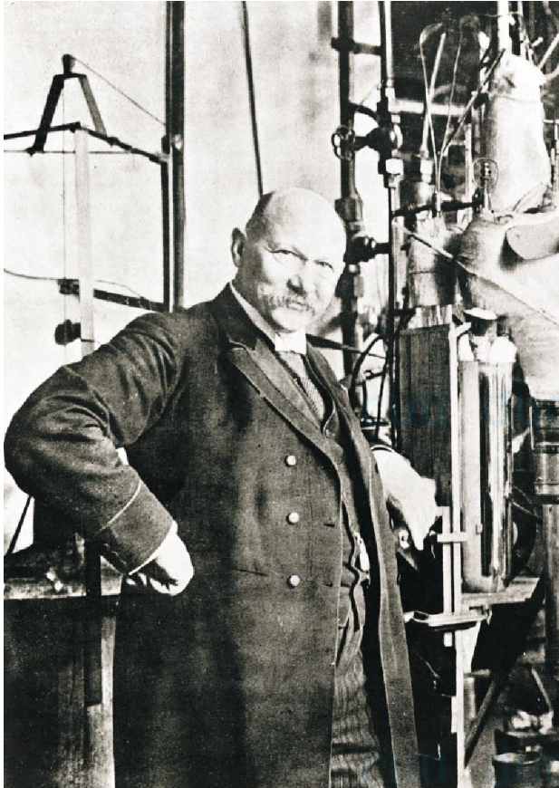
Kamerlingh Onnes, 1911
