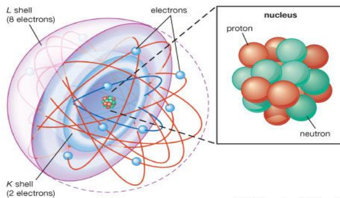
Hình 2.1. Mô hình cấu tạo nguyên tử
