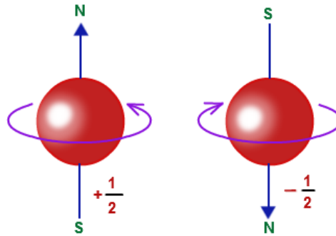
Hình 2.10: Trạng thái tự xoay của e
