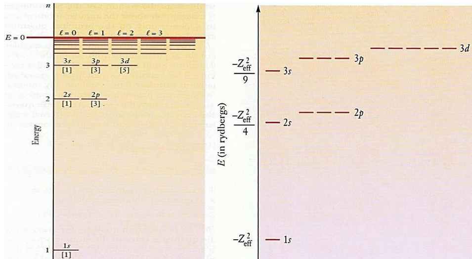
Hình 2-12: Biểu đồ mức năng lượng của nguyên tử H và nguyên tử đa e.
