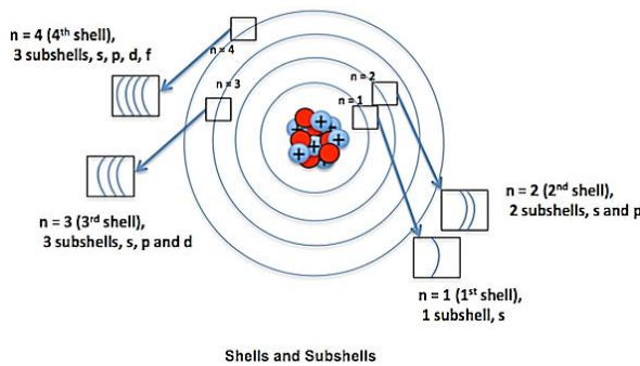
Hình 2.8: Các phân lớp e theo \ell
