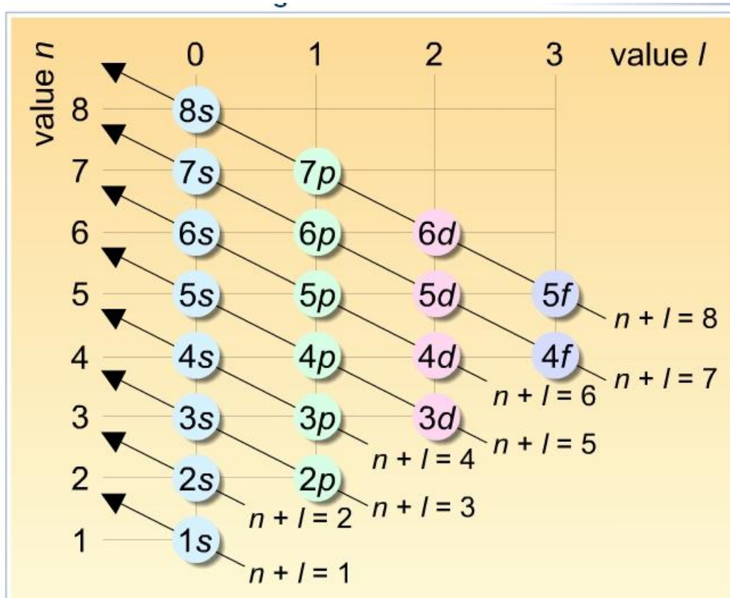
Hình 2.14: Quy tắc Klechkowski
