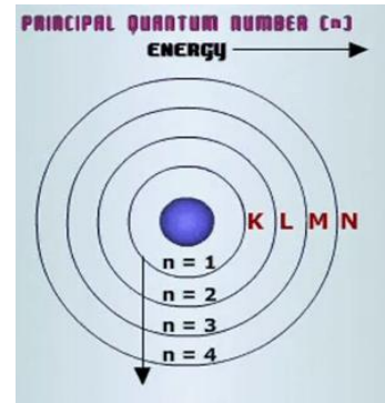
Hình 2.7: Các lớp e theo n
