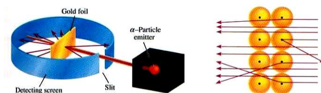
Hình 2.6: Thí nghiệm nhiễu xạ
