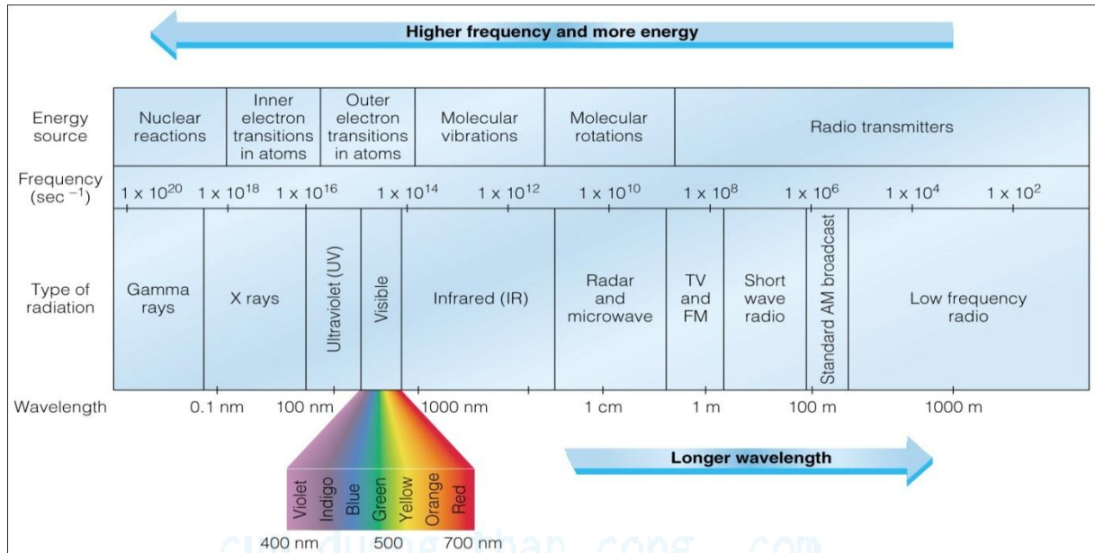
Hình 2.2. Phổ bức xạ điện từ (electromagnetic-spectrum)
