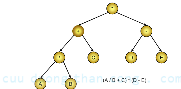
Hình 17: Cây biểu diễn biểu thức
