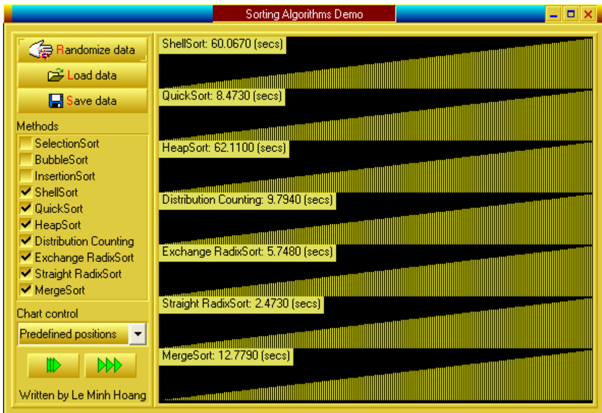
Hình 36: Cài đặt các thuật toán sắp xếp với dữ liệu lớn
