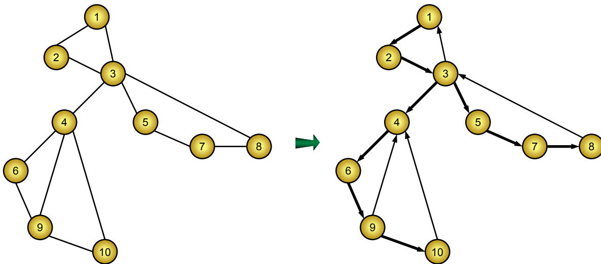
Hình 69: Phép định chiều DFS
