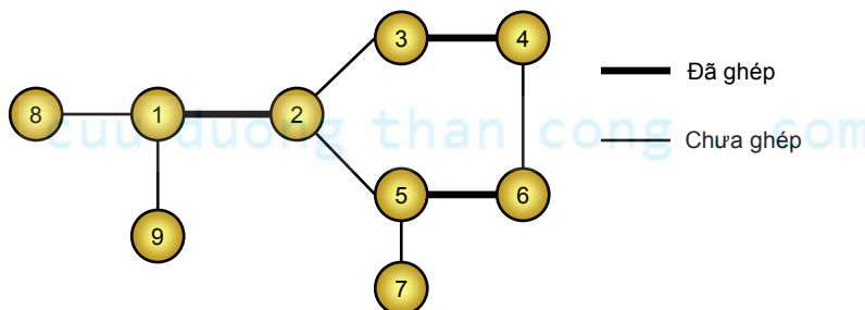
Hình 87: Đồ thị G và một bộ ghép M
