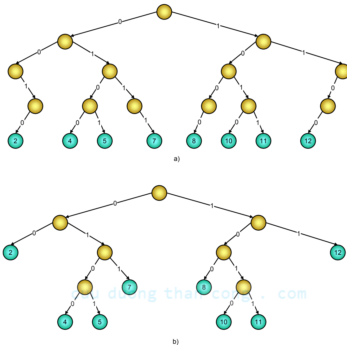
Hình 47: Cây tìm kiếm cơ số 2 a) và Trie tìm kiếm cơ số 2 b)
