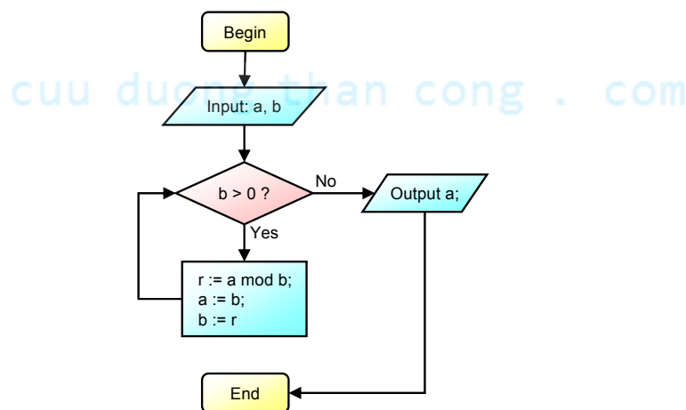
Hình 4: Lưu đồ thuật giải (Flowchart)
