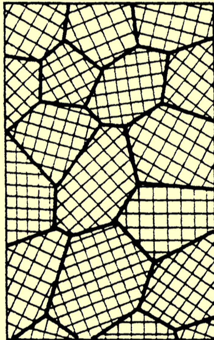
Cấu trúc đa tinh thể
