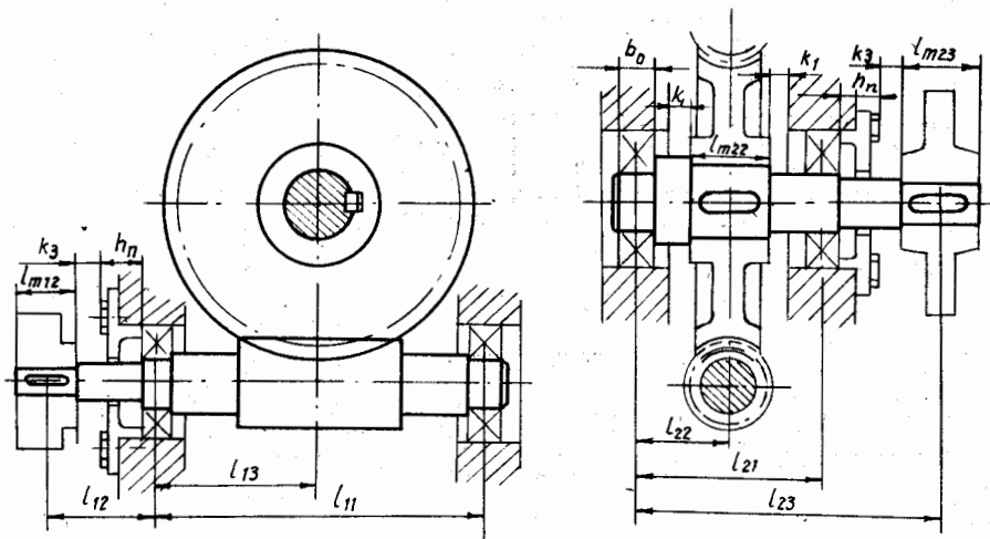
Hình 10.11. Sơ đồ tính khoảng cách đối với hộp giảm tốc trục vít
