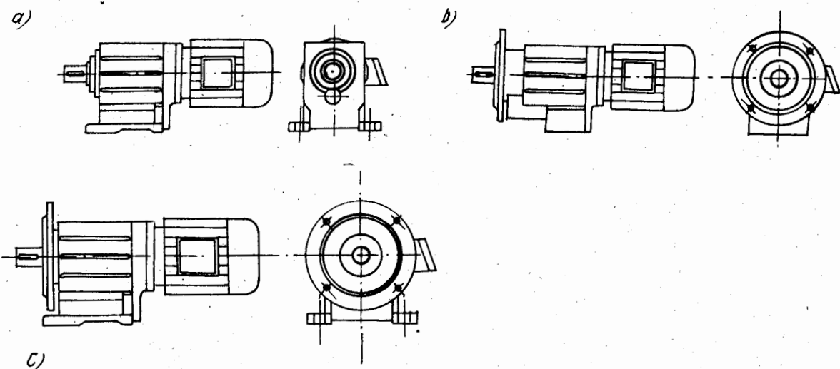
Hình 3.15. Các phương án lắp đặt động cơ - hộp giảm tốc
