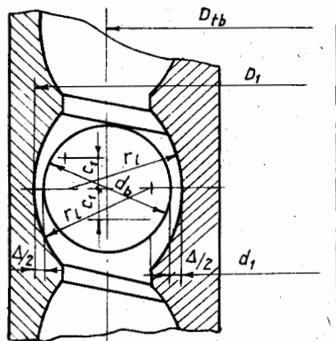
Hình 8.9. Các thông số của truyền động vít bi
