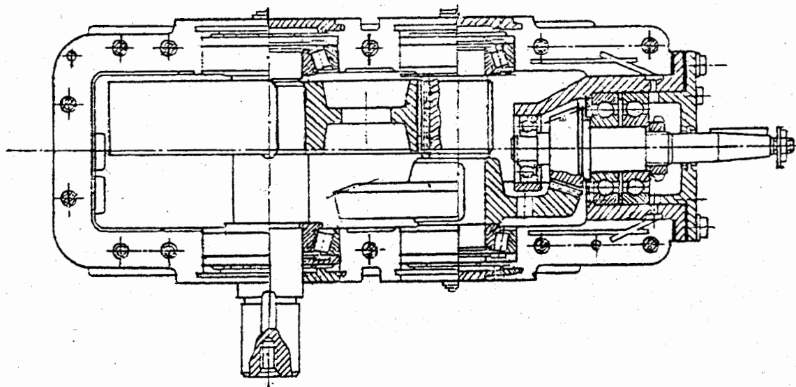
Hình 3.8. Hộp giảm tốc bánh răng côn - trụ với bánh răng côn không lắp chia
