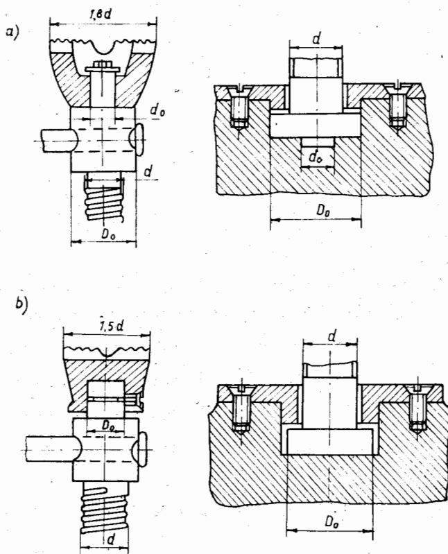
Hình 8.4. Kết cấu gối tì
