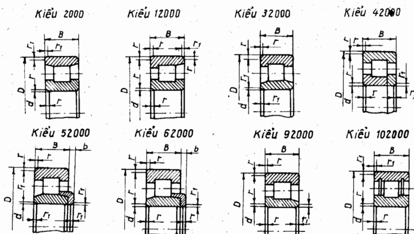
BẢNG P2.8 : Ổ ĐUA TRỤ NGẮN ĐỒ (THEO GOST 8328-75)
