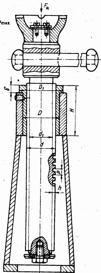
Hình 8.11. Kích vít
