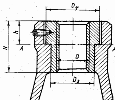
Hình 8.6. Đại ốc ghép
