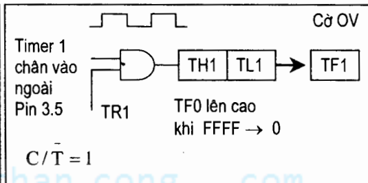
Hình 9.6. Timer 1, chân vào ngoài (Mode 1)
