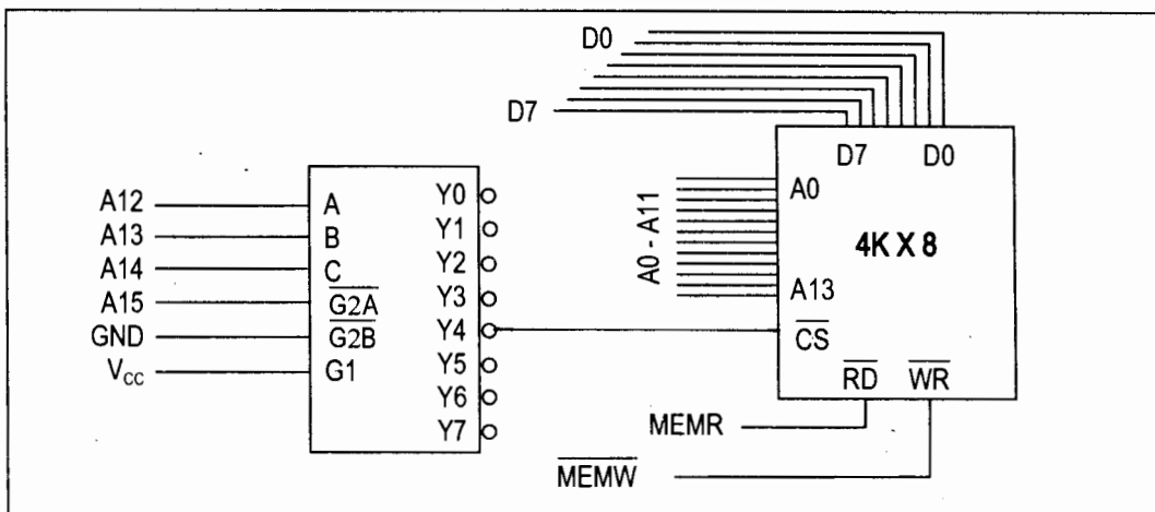
Hình 14.6. Mạch 74LS138 làm mạch giải mã
