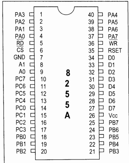
Hình 15.1. Chip 8255
