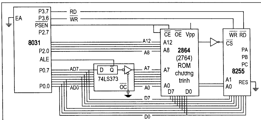
Hình 15.8. Nối ghép 8031 với 8255 và ROM chương trình ngoài
