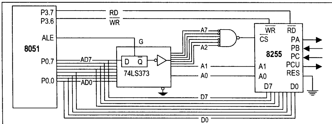
Hình 15.6. Nối ghép 8051 với 8255 ở ví dụ 15.4
