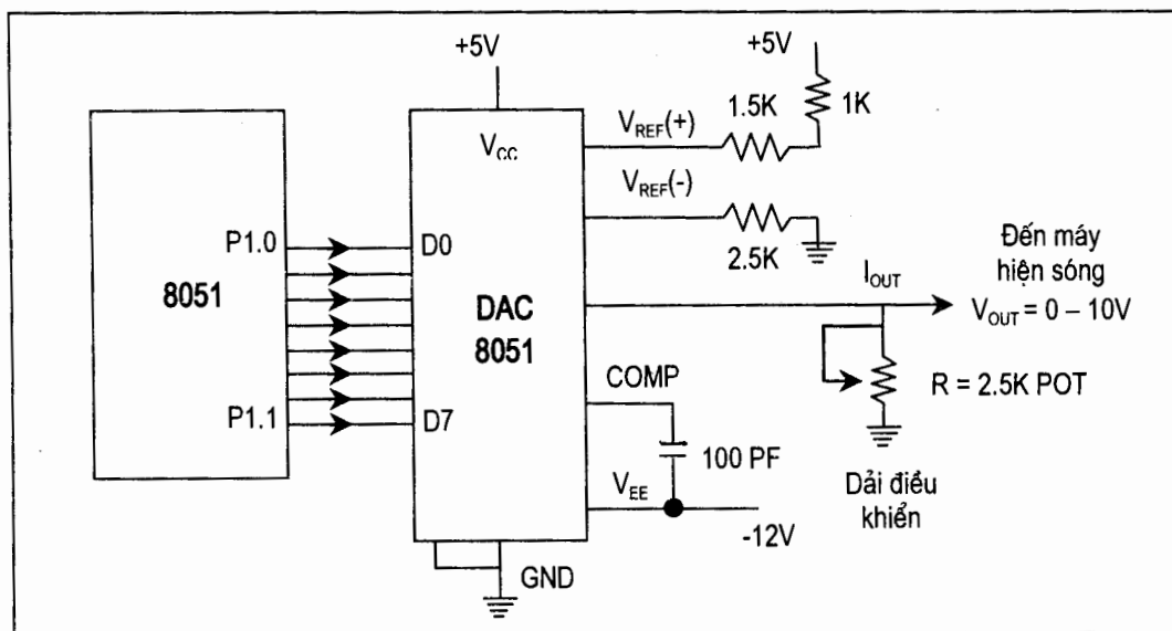
Hình 13.7. Nối ghép 8051 với DAC808 cong . com
