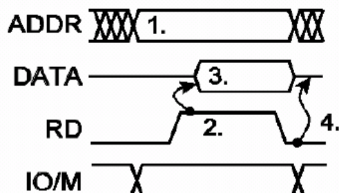
Hình 1.35 Thí dụ chu kỳ đọc bus.
