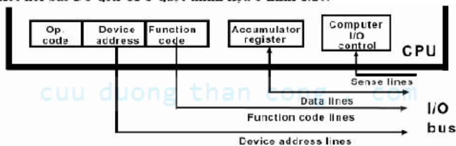
Hình 1.20 Kết nối bus I/O đến CPU
