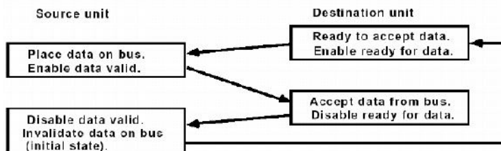
(c) Trình tự các sự kiện
