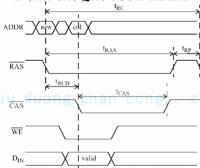
Hình 1.49 Định thì ghi DRAM
