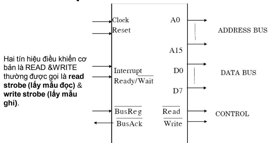
Hình 1.12 Các tín hiệu vi xử lý cơ bản.
