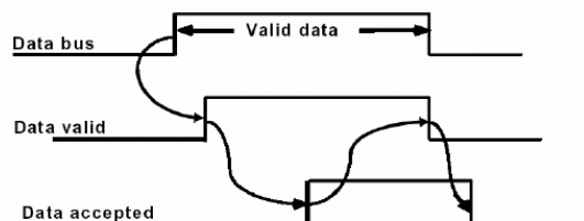
(b) Giãn đồ định thời
