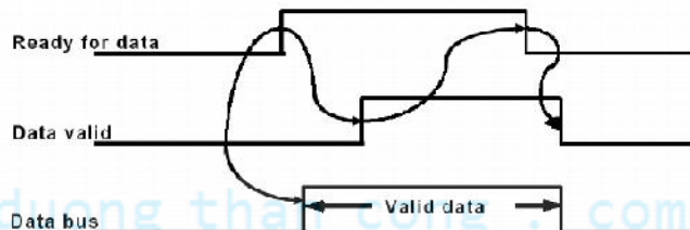
(b) Giãn đồ định thời
