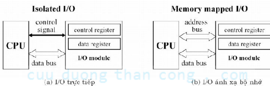
Hình 1.22 I/O trực tiếp và I/O ánh xạ bộ nhớ
