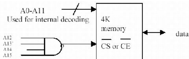
Hình 1.37 Dùng NAND để giải mã địa chỉ.
