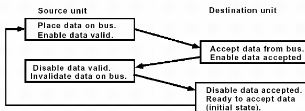
(c) Trình tự các sự kiện
