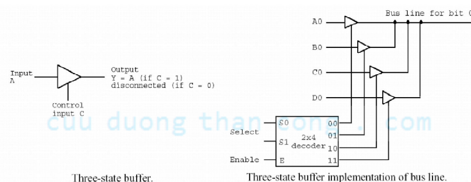
Hình 1.34 Thí dụ bus chung với bộ đệm 3 trạng thái.
