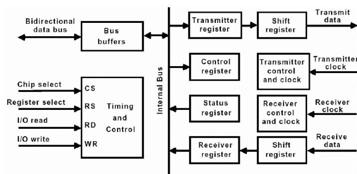
Hình 1.27 Sơ đồ khối một UART tiêu biểu.
