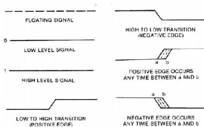
Hình 1.40 Các biểu diễn giản đồ định thời cho một tín hiệu. Các đường ngang kết hợp với các đường chéo chỉ những chuyển tiếp trong các mức logic.
