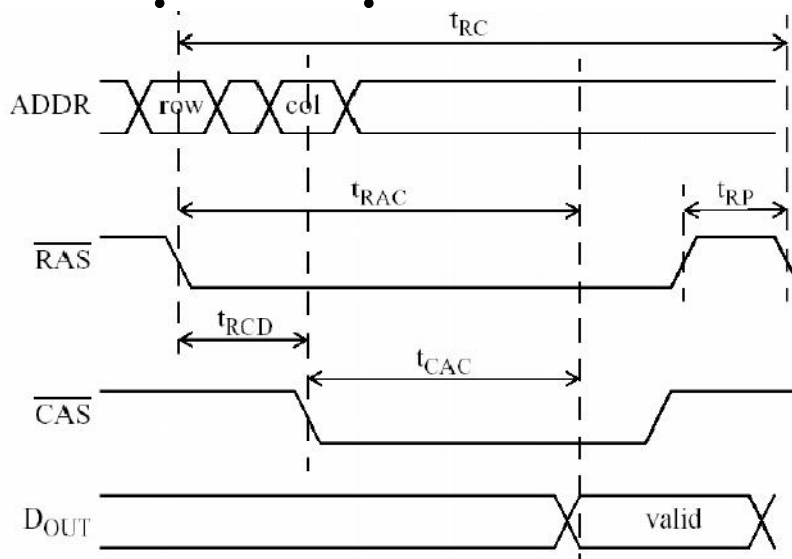
Hình 1.48 Định thì đọc DRAM
