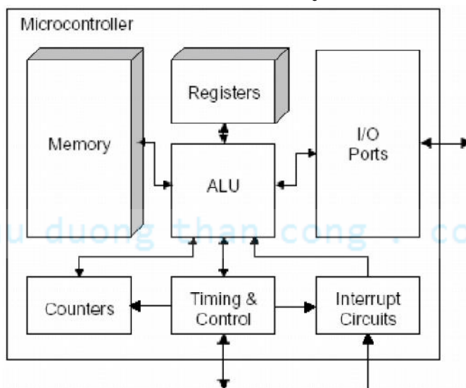
Hình 1.54 Sơ đồ khối một MCU
