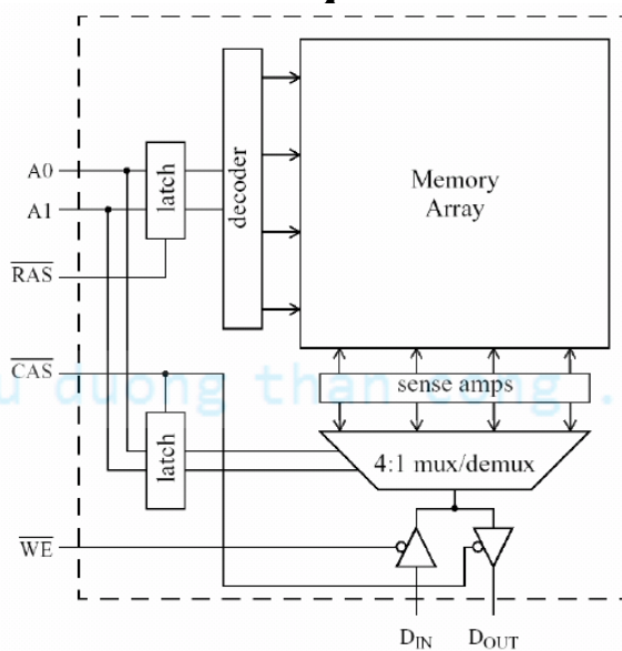
Hình 1.47 Sơ đồ khối của DRAM 4 x 1.
