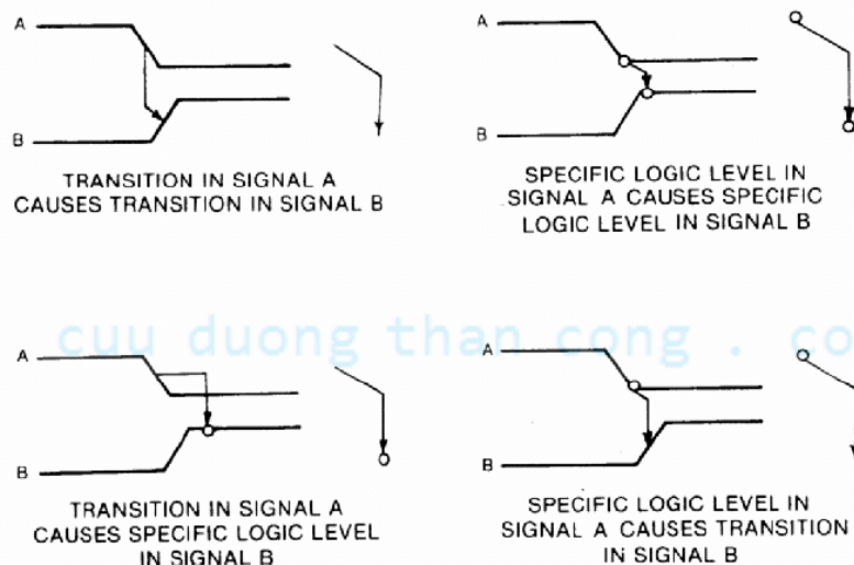
Hình 1.41 Các giản đồ định thời. Các quy ước cho cặp tín hiệu minh họa 4 cách mà một tín hiệu có thể cho phép hoặc kích một tín hiệu khác.
