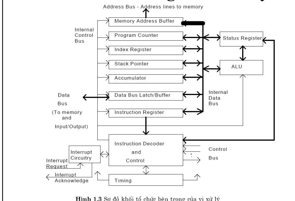
Hình 1.3 Sơ đồ khối tổ chức bên trong của vi xử lý
