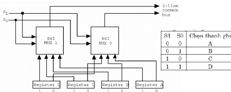
Hình 1.33 Thí dụ Bus dồn kênh có 2 đường.
