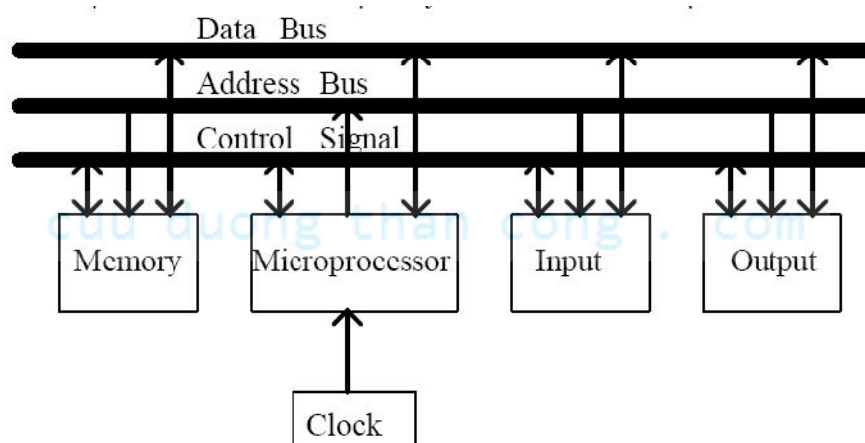
Hình 1.2 Sơ đồ khối của máy vi tính
