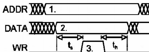
Hình 1.36 Thí dụ chu kỳ ghi bus.
