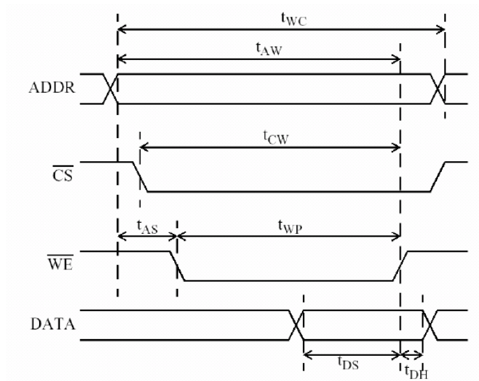
Hình 1.46 Định thì ghi bộ nhớ tiêu biểu.
