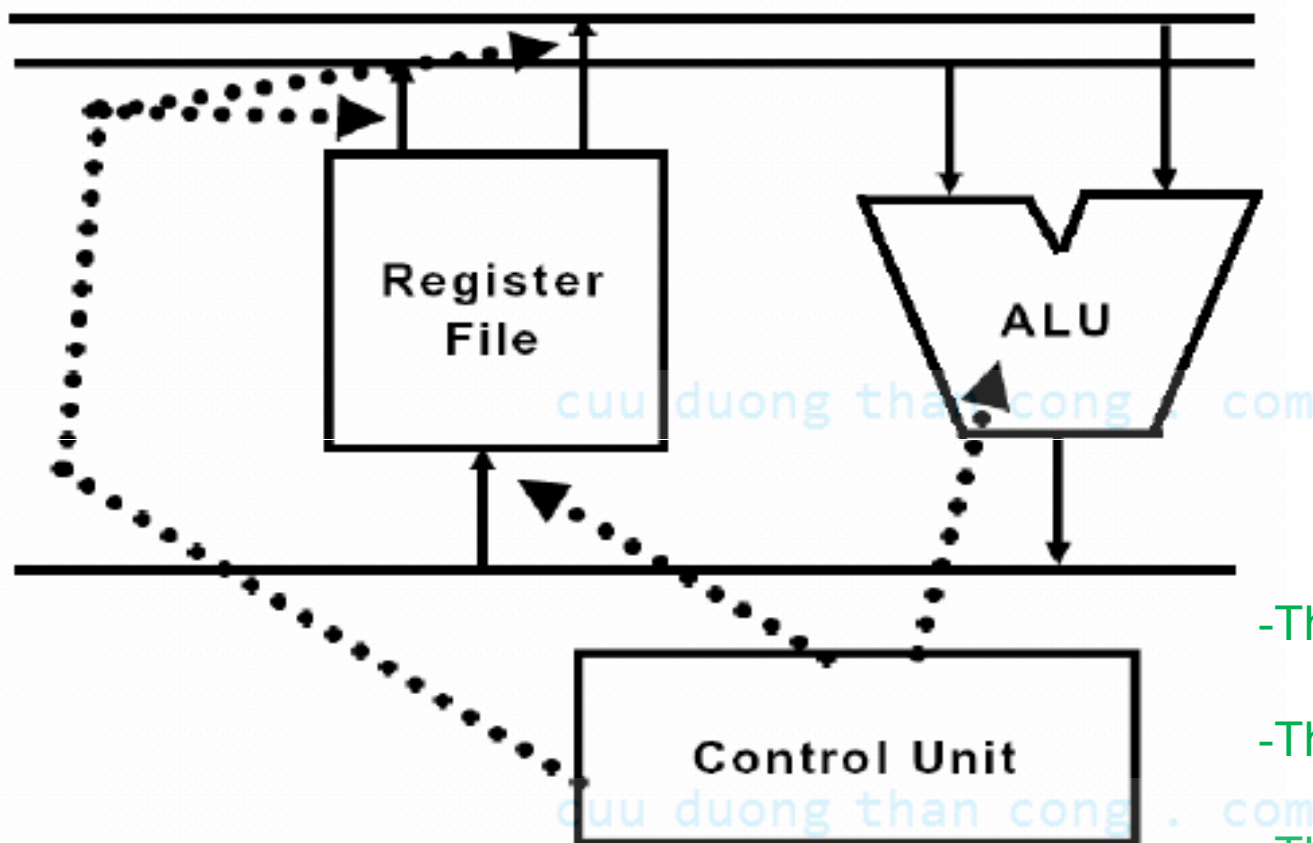
Hình 1.13 Các thành phần chính của CPU
