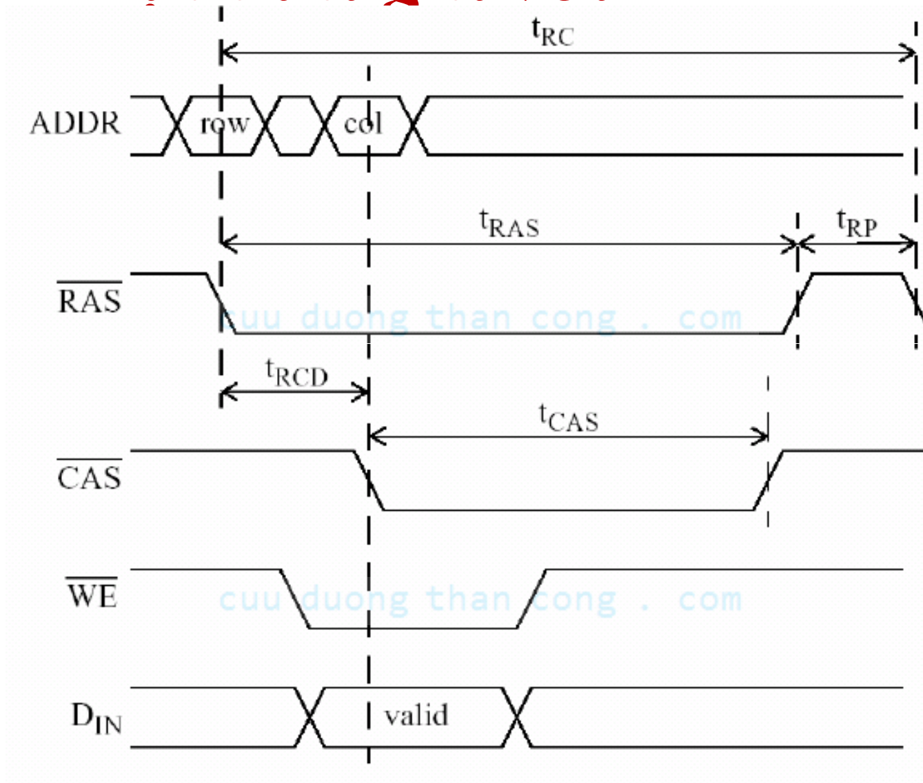
Hình 1.49 Định thời ghi DRAM
