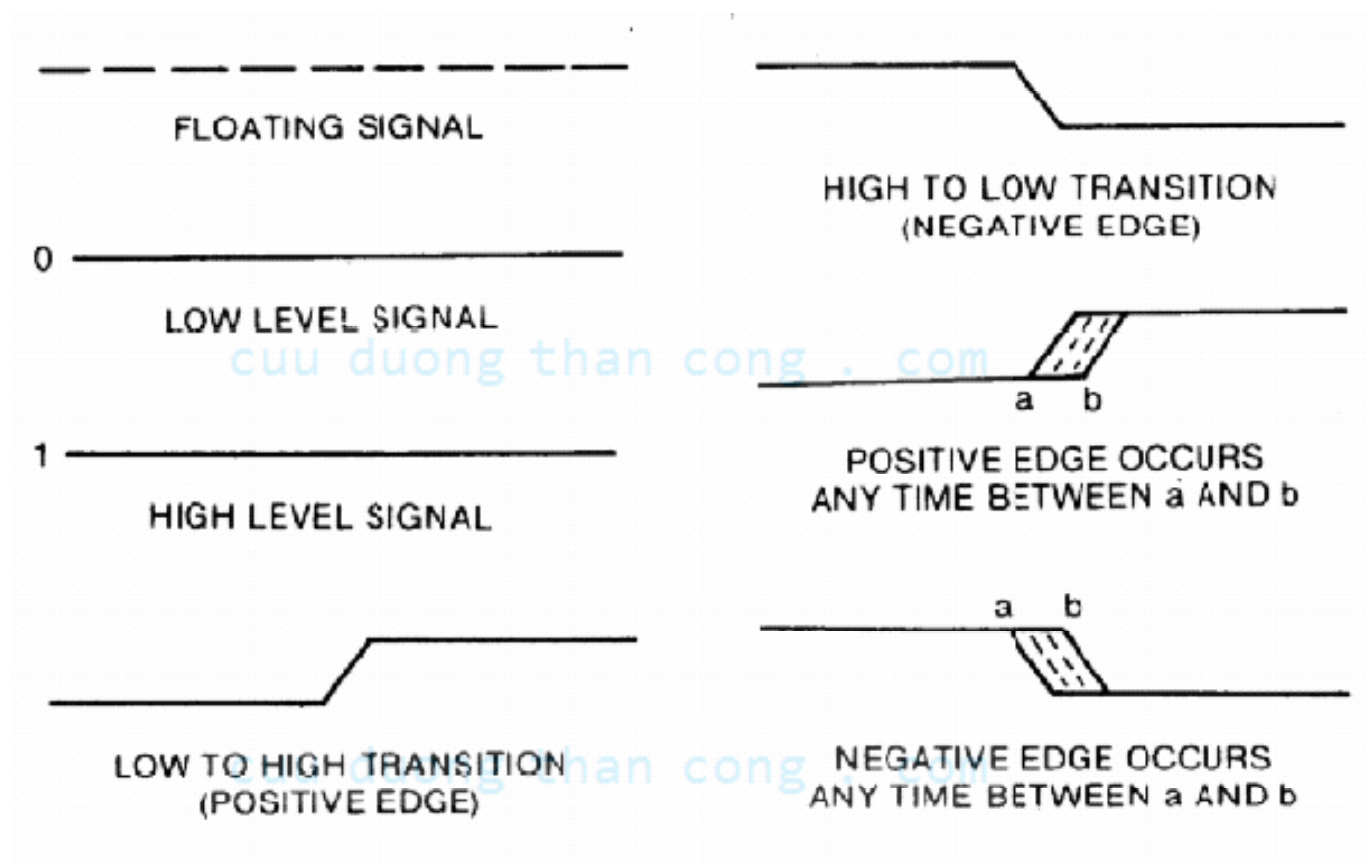
Hình 1.40 Các biểu diễn giản đồ định thì cho một tín hiệu. Các đường ngang kết hợp với các đường chéo chỉ những chuyển tiếp trong các mức logic.
