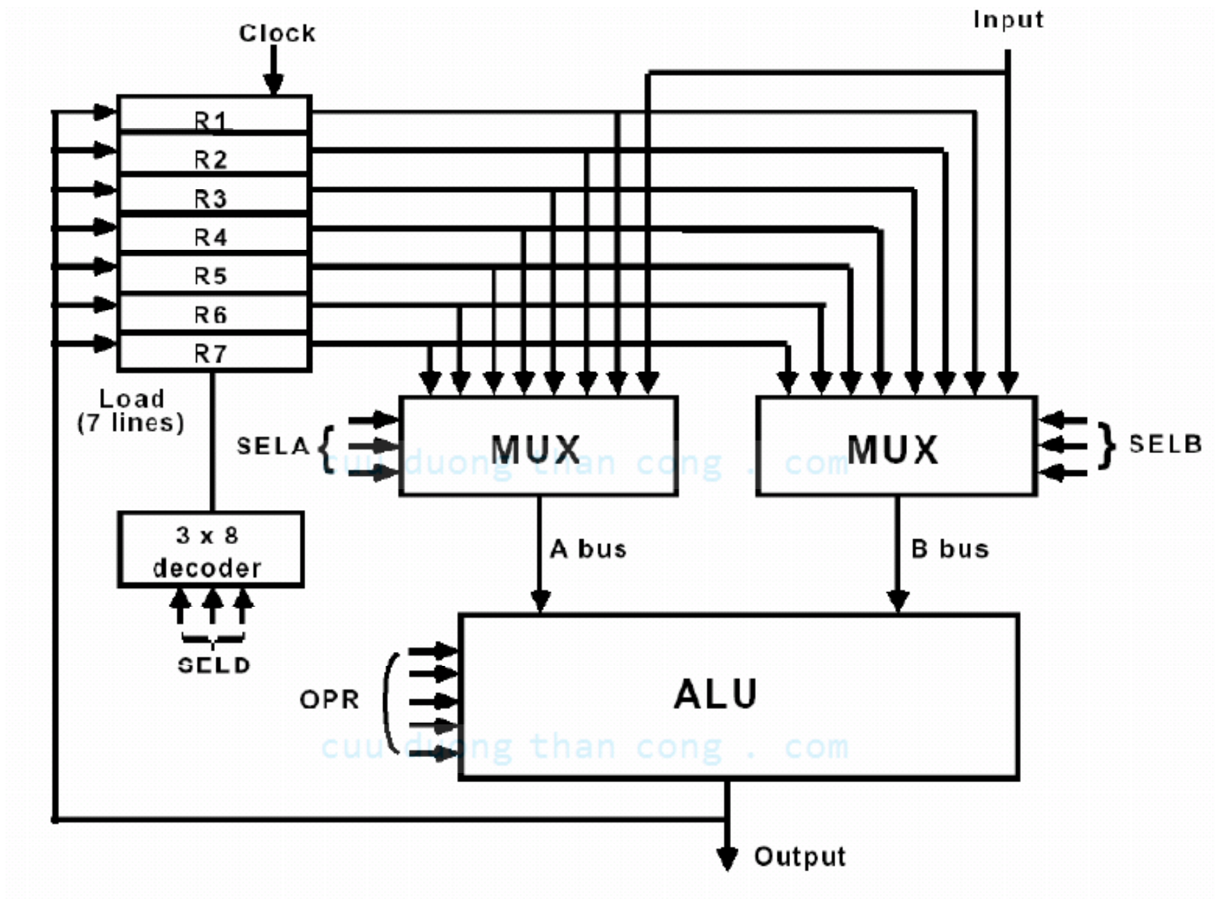
Hình 1.14 Tổ chức các thành ghi
