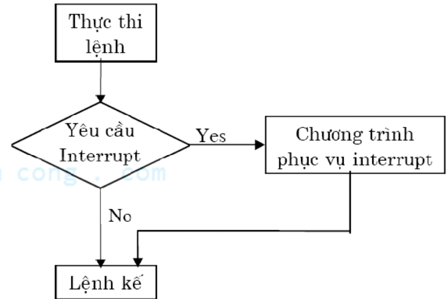
Hình 1.31 Logic ngắt.
