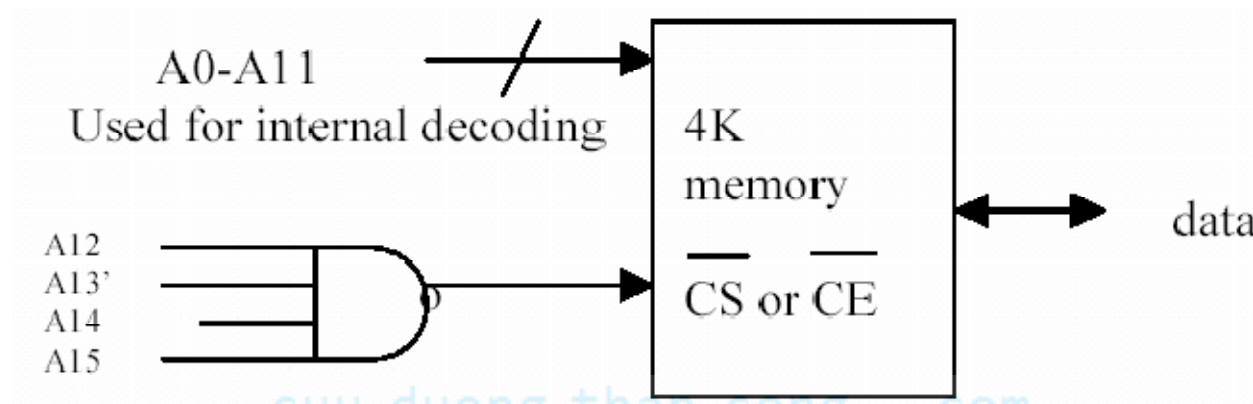
Hình 1.37 Dùng NAND để giải mã địa chỉ.
