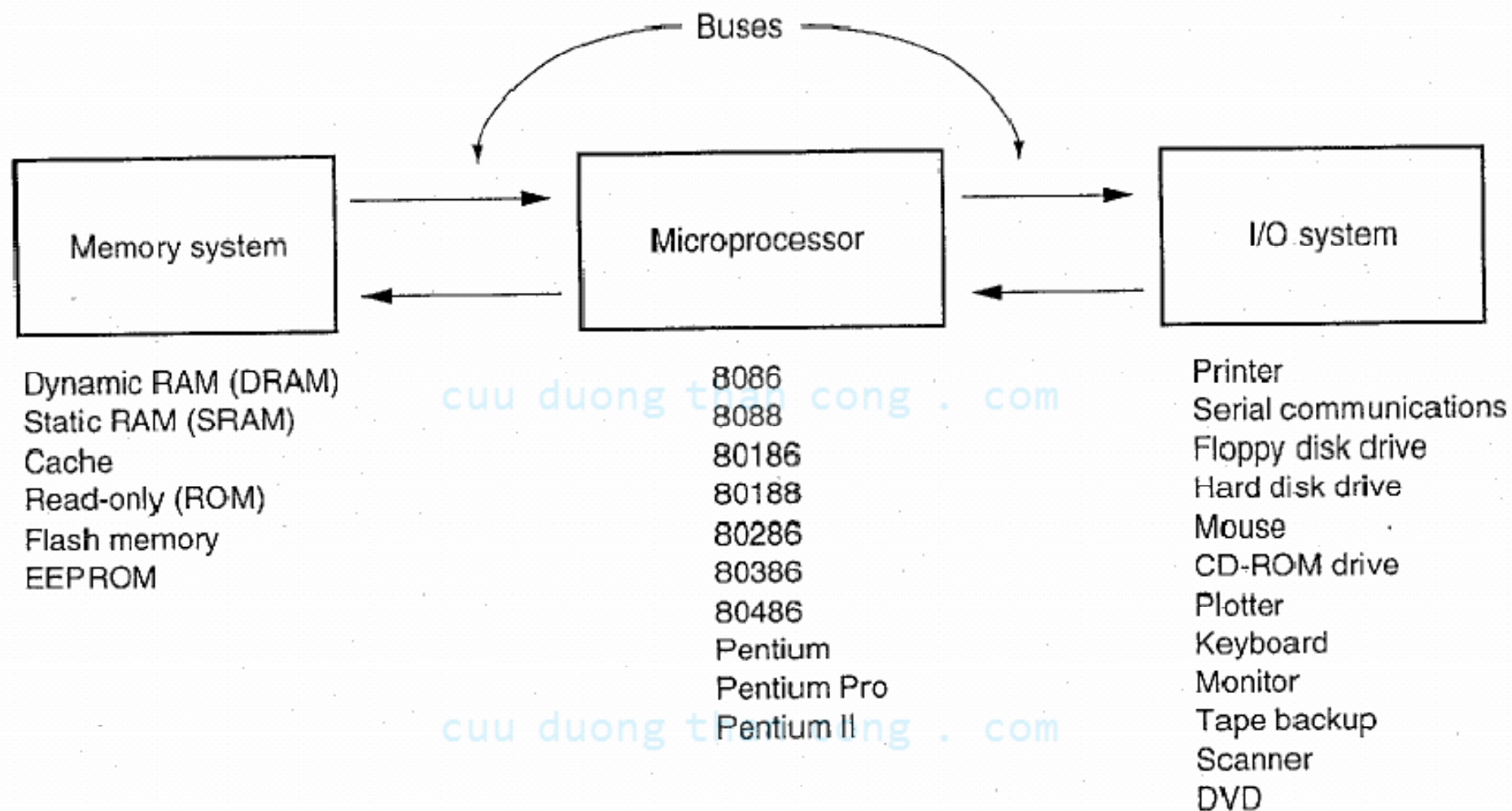
Hình 1.7 Các hệ thống máy tính dựa trên vi xử lý.
