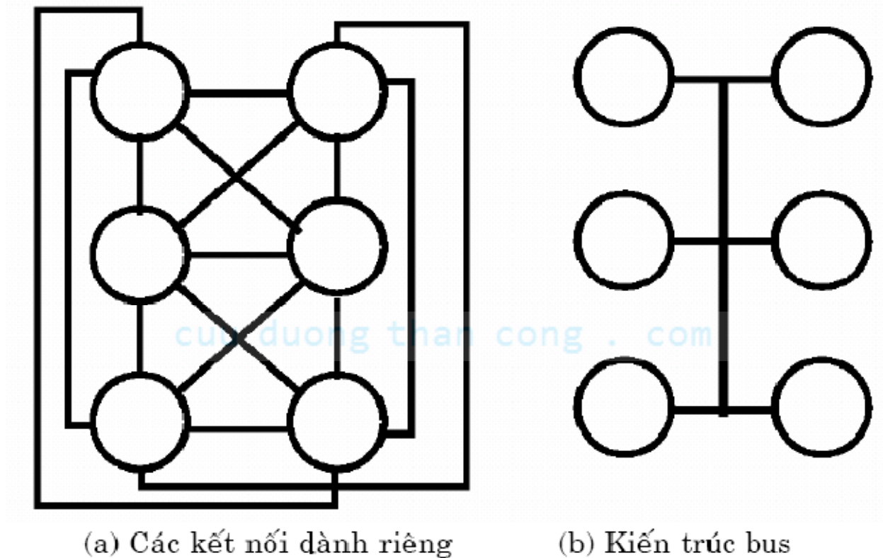
Hình 1.32 Các kết nối nhiều điểm khi không có bus và có bus.
