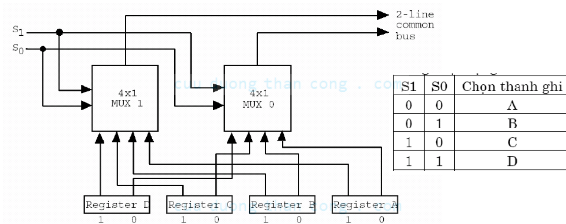
Hình 1.33 Thí dụ Bus dồn kênh có 2 đường.
