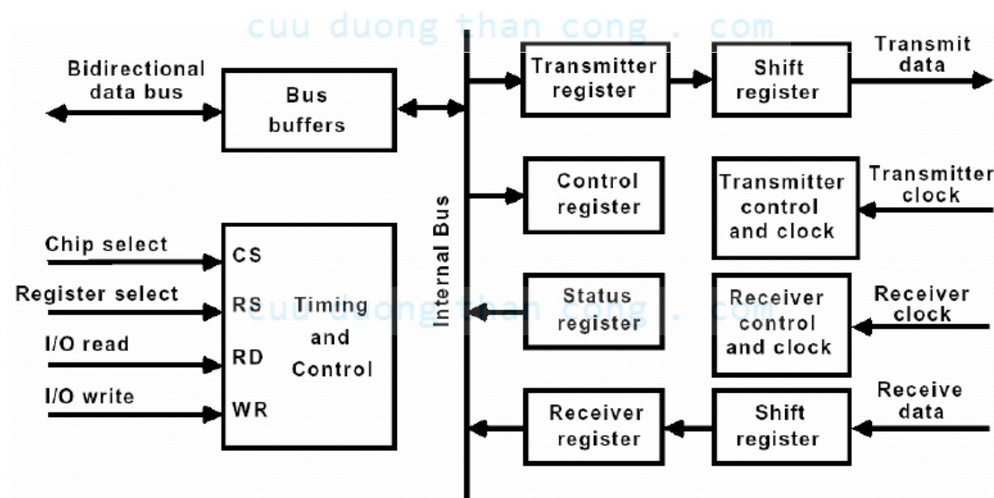
Hình 1.27 Sơ đồ khối một UART tiêu biểu.
