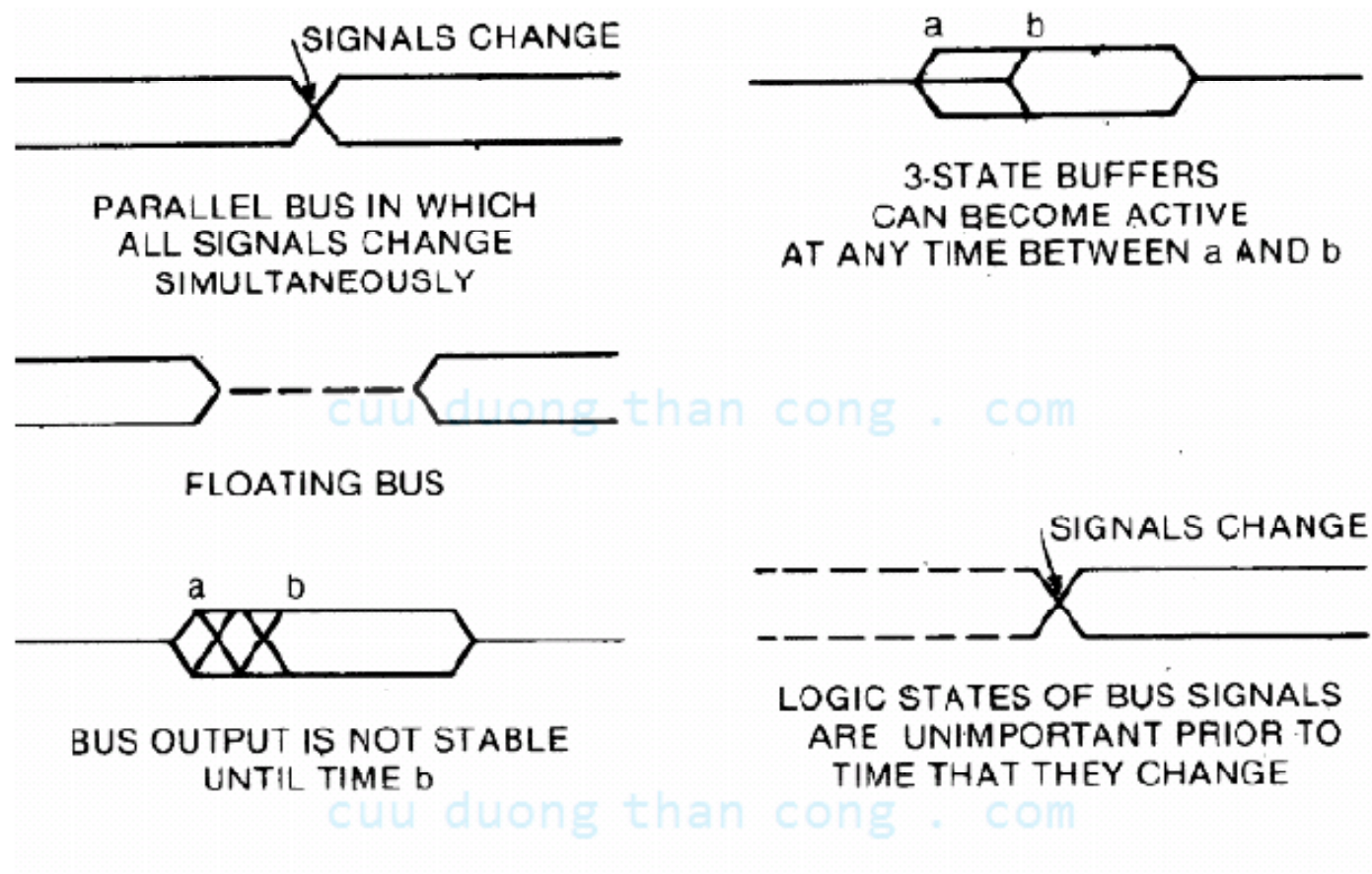
Hình 1.43 Các giản đồ định thì bus. Các biểu diễn minh họa 5 quy ước cho bus với 2 hay nhiều tín hiệu
