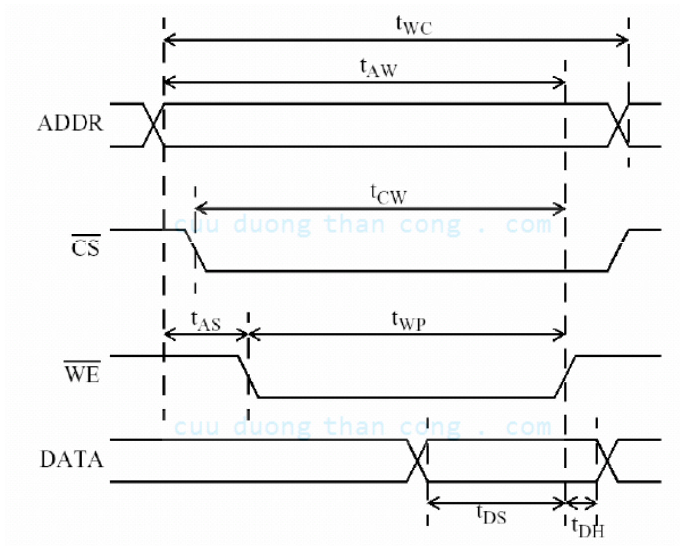
Hình 1.46 Định thì ghi bộ nhớ tiêu biểu.
