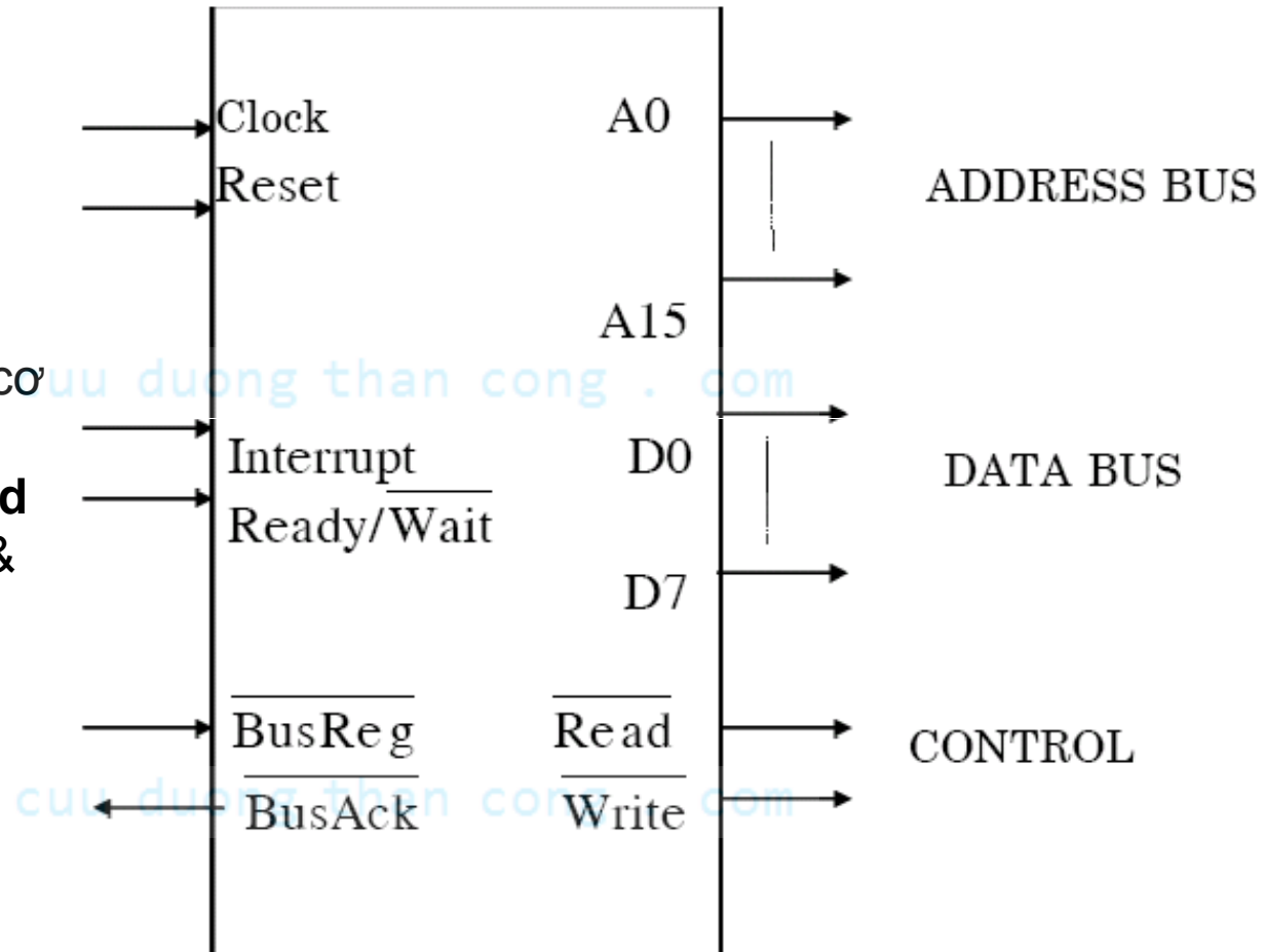
Hình 1.12 Các tín hiệu vi xử lý cơ bản.
