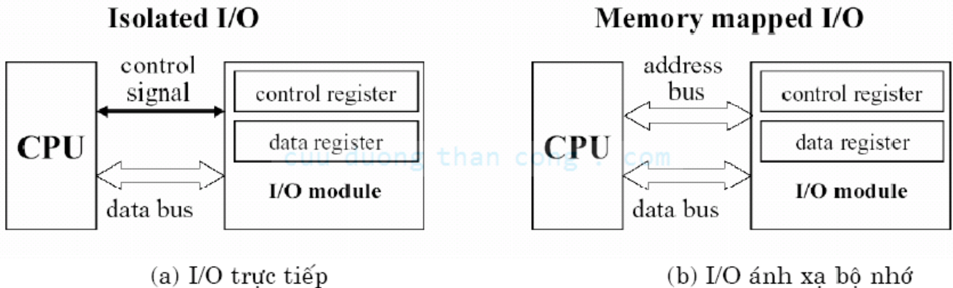
Hình 1.22 I/O trực tiếp và I/O ánh xạ bộ nhớ
