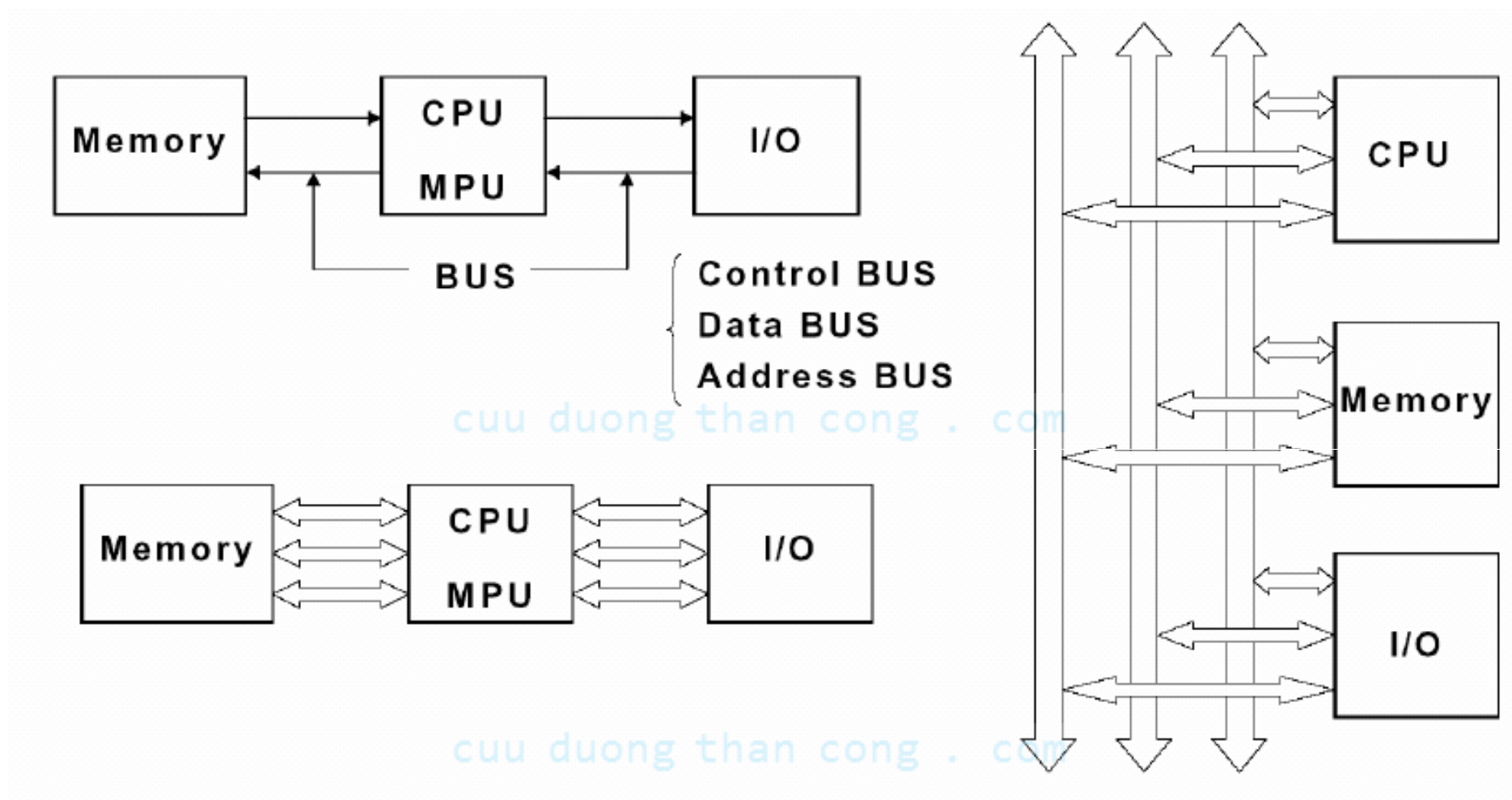
Hình 1.5 Các kết nối cơ bản với vi xử lý
