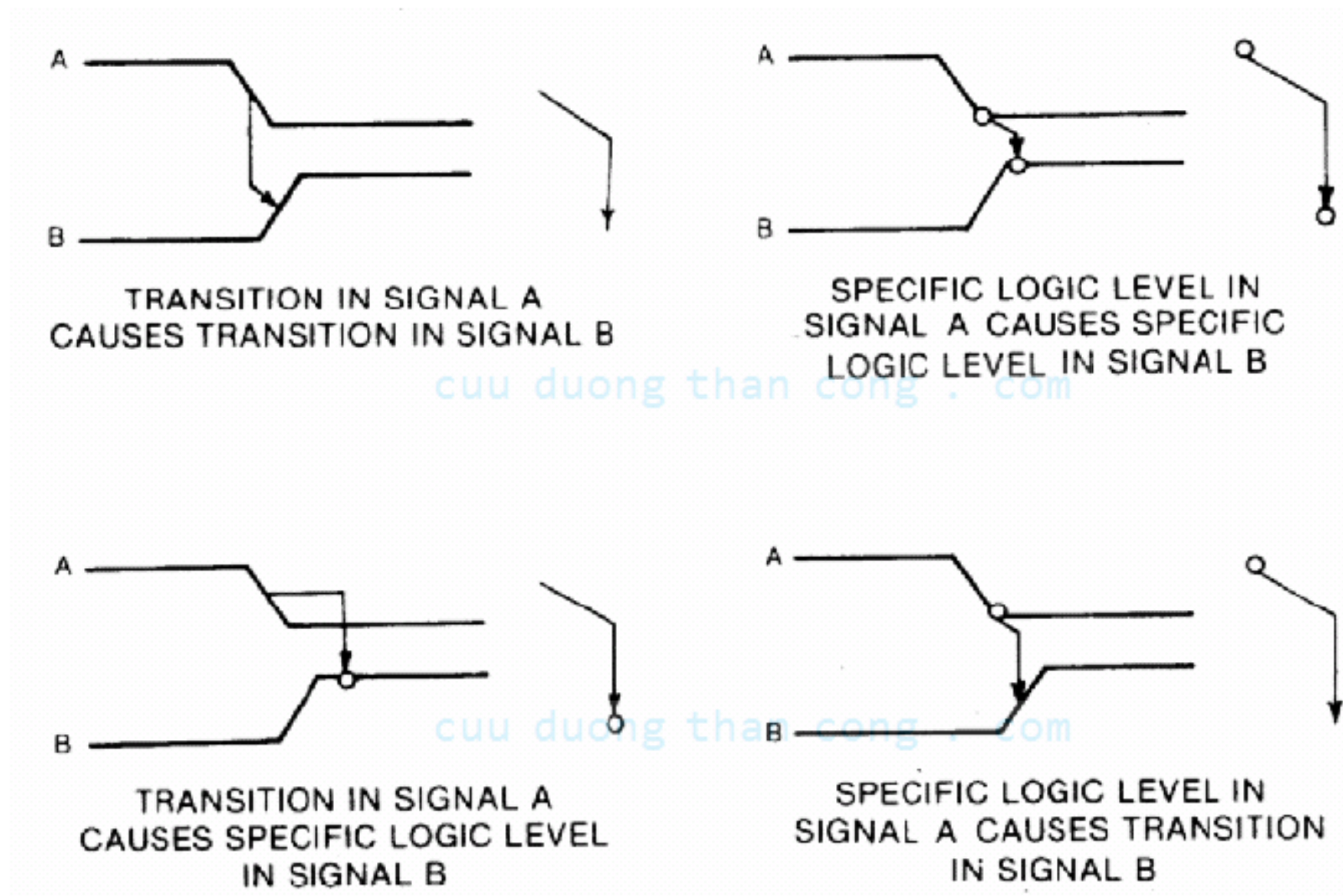
Hình 1.41 Các giản đồ định thì. Các quy ước cho cặp tín hiệu minh họa 4 cách mà một tín hiệu có thể cho phép hoặc kích một tín hiệu khác.
