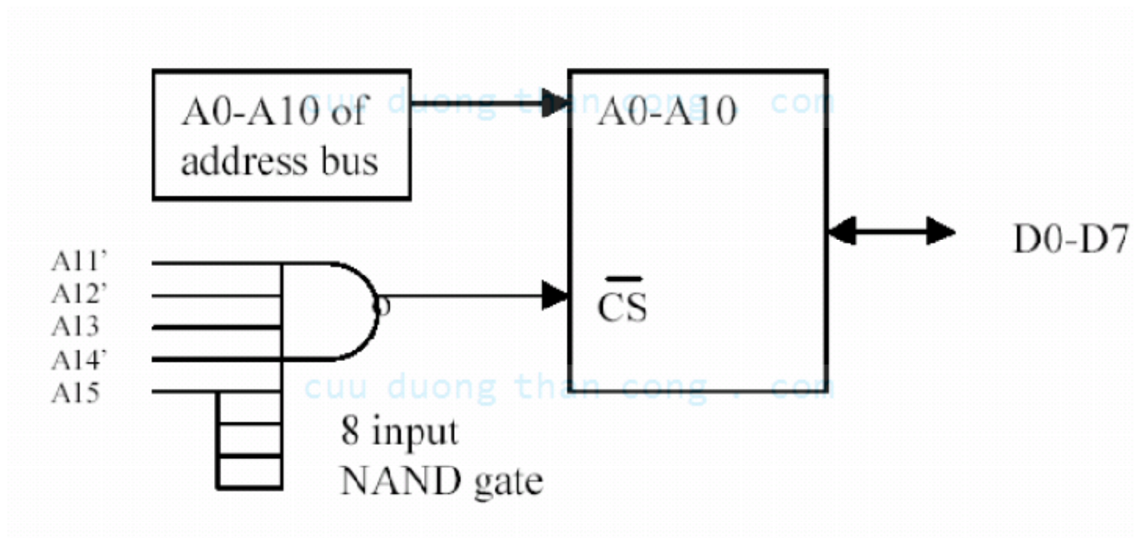
Hình 1.38 Cài đặt giải mã địa chỉ bằng NAND.
