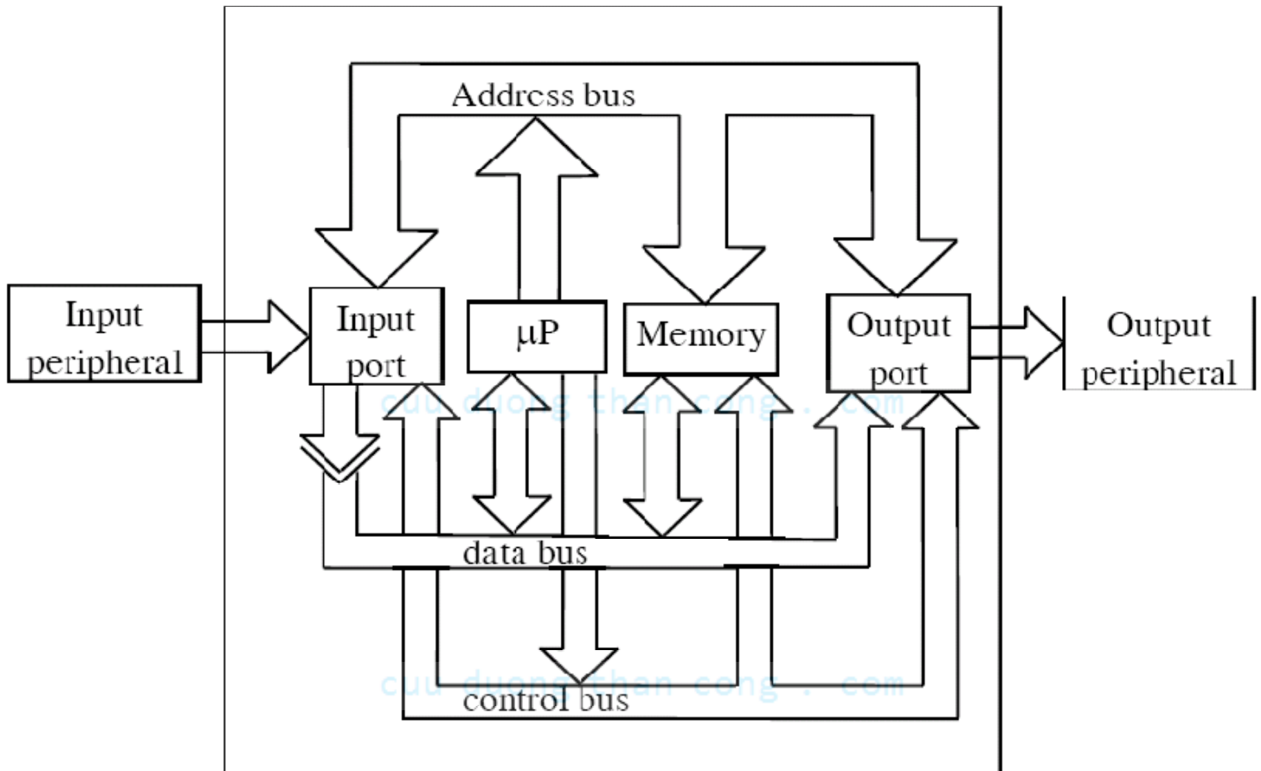
Hình 1.9 Sơ đồ khối một hệ thống vi xử lý cơ bản.
