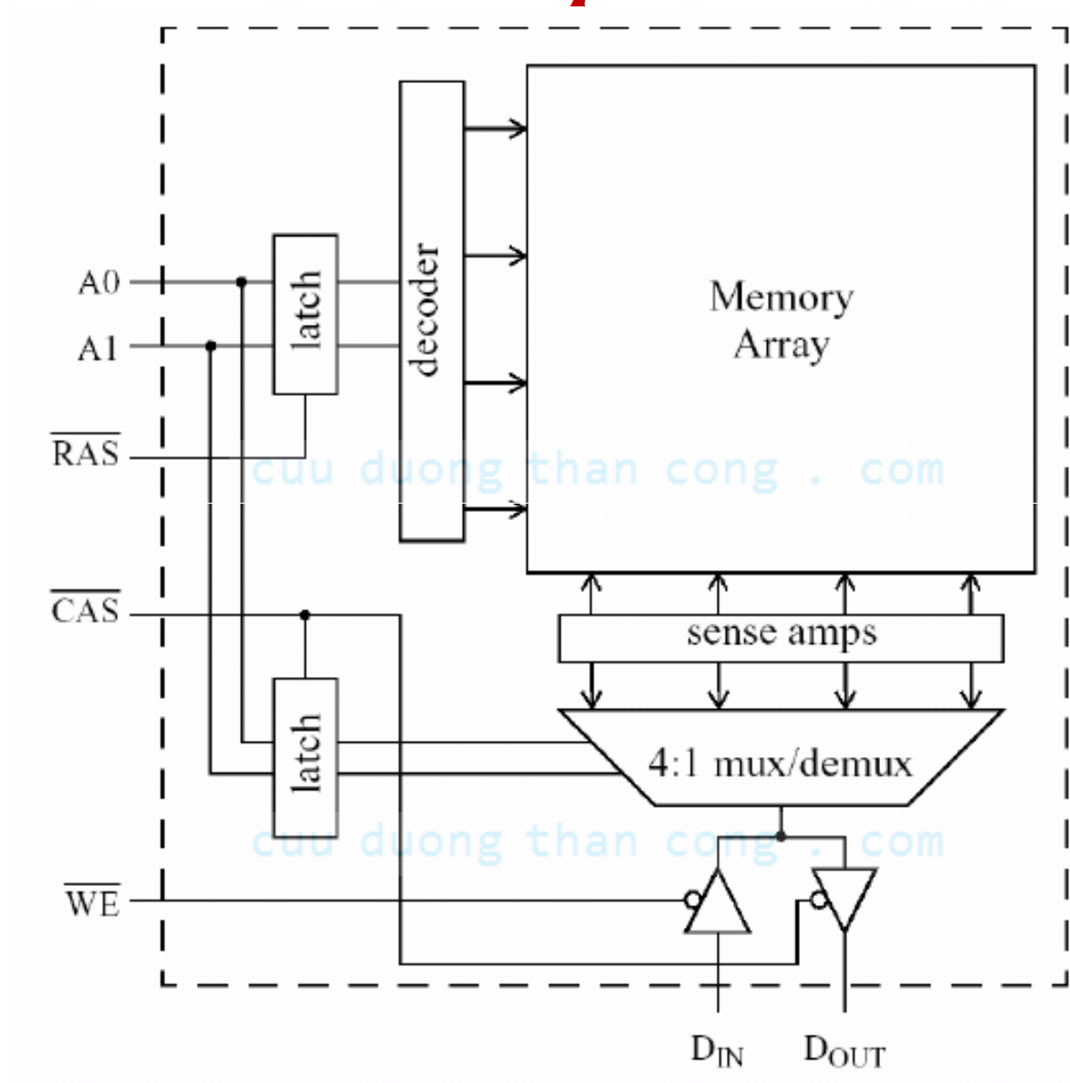
Hình 1.47 Sơ đồ khối của DRAM 4 x 1.
