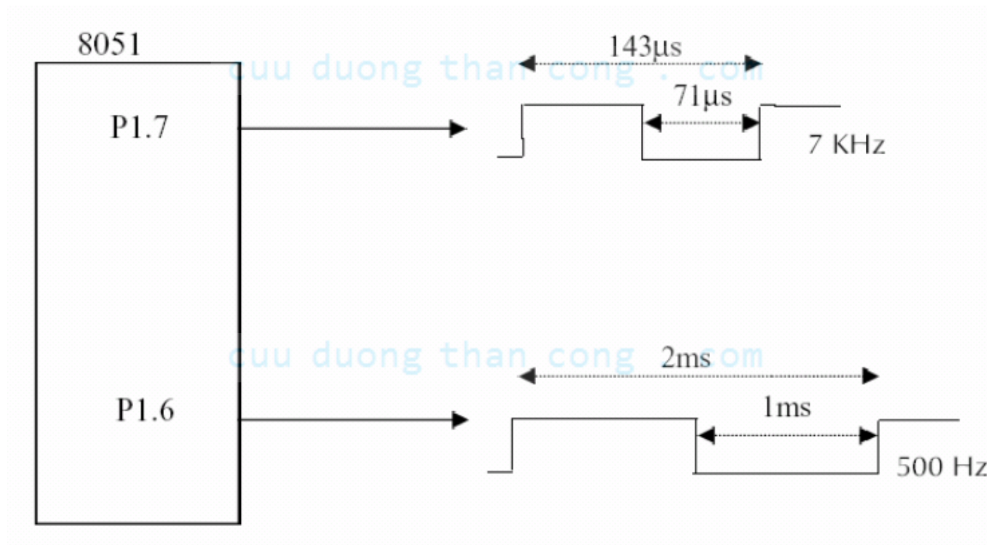
Hình 3.39 Dạng sóng 7 KHz và 500 Hz.
