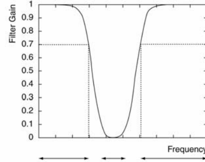
(d) Band Stop Filter
