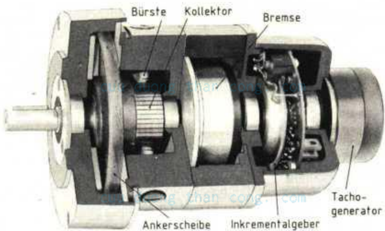
Bild 3: Scheibenläufermotor
