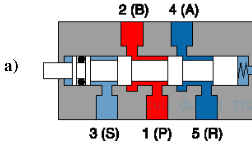
Hình 2.50 Cấu tạo van 5/2 và kí hiệu
