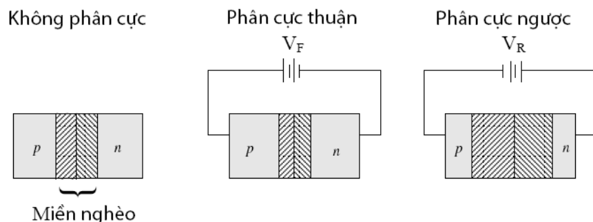
Hình 4.3 Các phân cực có thể có ở chuyển tiếp PN
