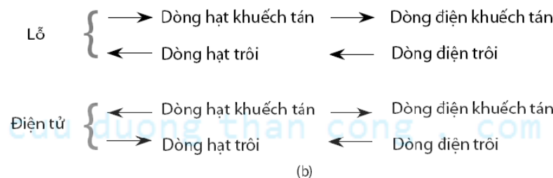
Hình 4.2 Chuyển tiếp PN chưa có phân cực
