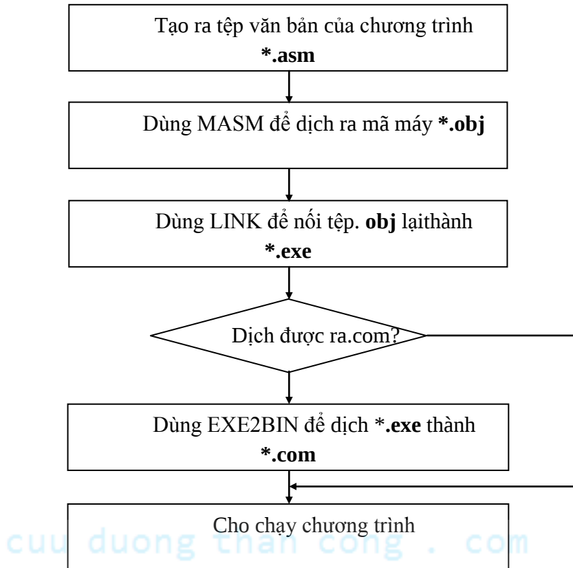
Hình 3-3. Các bước để tạo ra và chạy chương trình hợp ngữ
