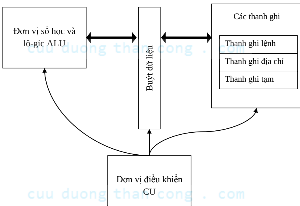
Hình 1-2. Sơ đồ khối chức năng vi xử lý
