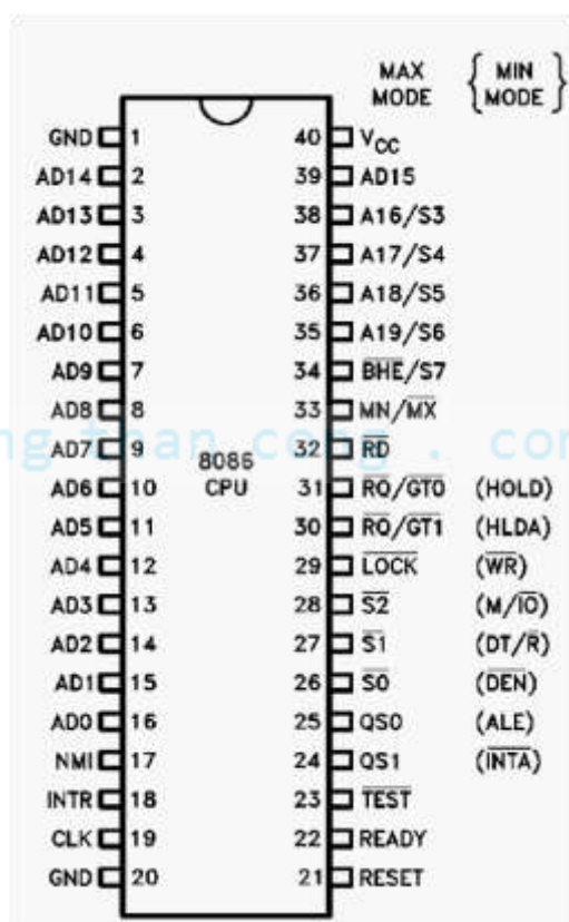
Hình 4-1. Tín hiệu 8086
