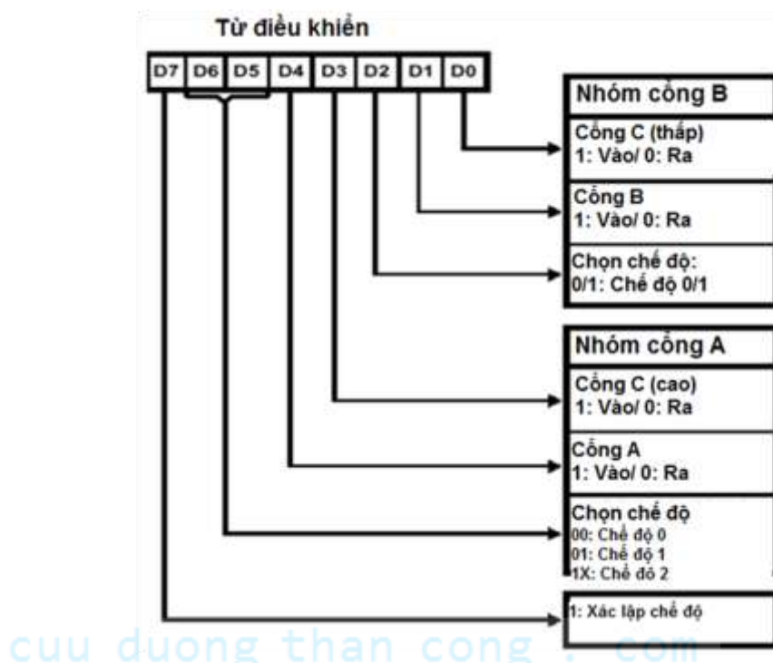
Hình 4-25. Thanh ghi điều khiển chế độ
