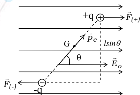
Hình 7-6. Lưỡng cực điện trong điện trường đều
