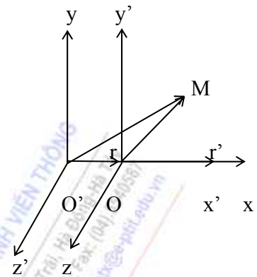
Hình 2-8 Để tổng hợp vận tốc và gia tốc
