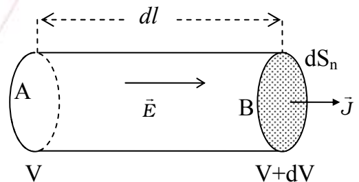
Hình 10-7. Để thiết lập dạng vi phân của định luật Ohm.
