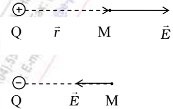
Hình 7-3. Cường độ điện trường gây bởi một điện tích điểm
