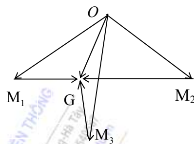
Hình 4-2 Để xác định khối tâm của hệ chất điểm
