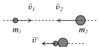
Hình 3-9 Va chạm mềm giữa hai vật
