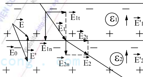
Hình 9-4. Sự không liên tục của đường sức điện trường
