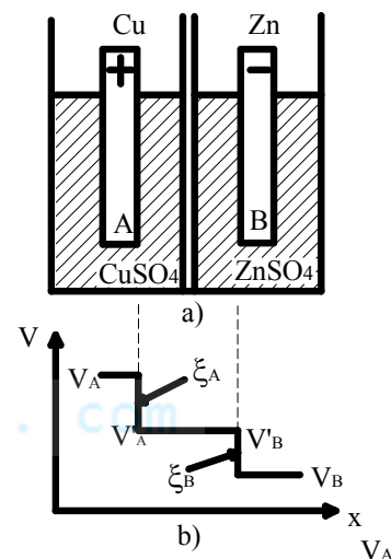
Hình 10-9. a) Cấu tạo pin Đaniell b) Sơ đồ phân bố điện thế trong pin
