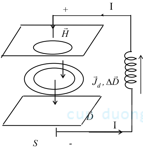
Hình 13-5 Dòng dịch nối tiếp dòng điện dẫn trong mạch kín khi tụ nạp điện
