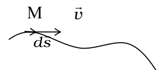
Hình.1-3 Định nghĩa vector vận tốc
