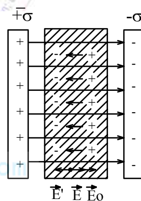
Hình 9-3 Điện trường
