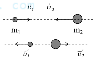
Hình 3-8 Va chạm đàn hồi giữa hai vật
