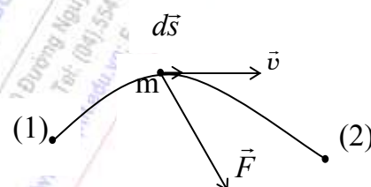
Hình 3-4. Minh họa xác định công của trường lực thể
