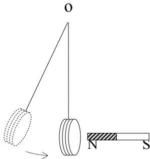
Hình 11-2 Nam châm tác dụng lên dòng điện
